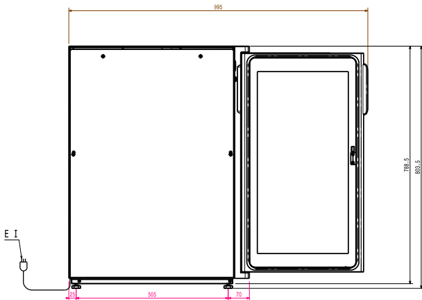
Zij aanzicht
